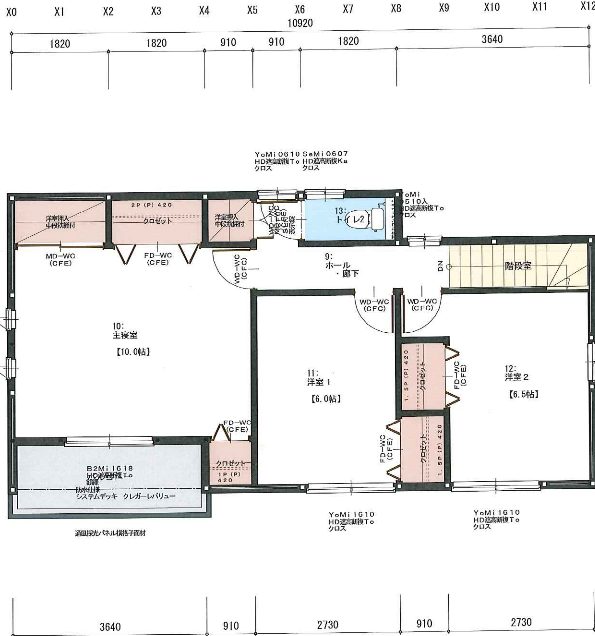
ー 2 階 平 面 図 ー
