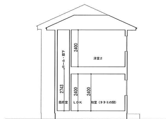
断 面 X - X
