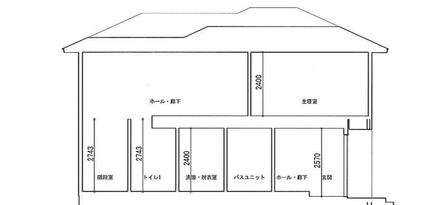
断 面 Y - Y
